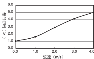
D6F-W04A1
