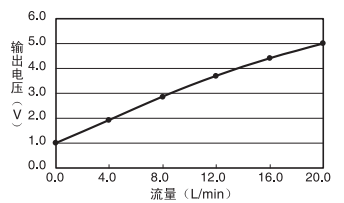
D6F-20A5-000
