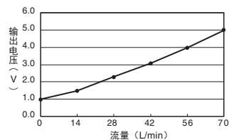
D6F-70AB71-000
