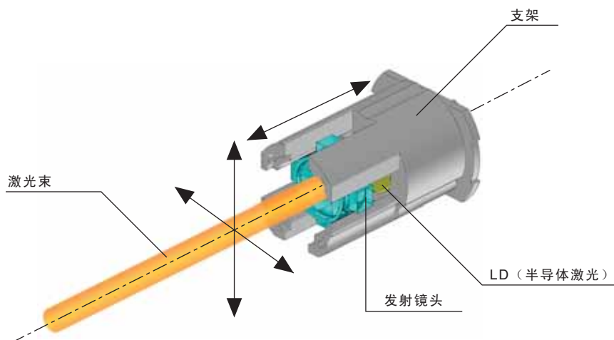
激光模块概念图
